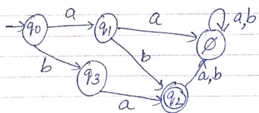
DFA
